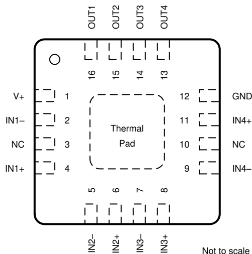
注: 露出サーマル・パッドは GND ピンに直接接続します。 図 4-6. RTE パッケージ 16 パッド WQFN (露出サーマル・パッド付き) 上面図
