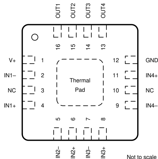
図 4-6. RTE パッケージ 16 パッド WQFN (露出サーマル・パッド付き) 上面図 注: 露出サーマル・パッドは GND ピンに直接接続します。
