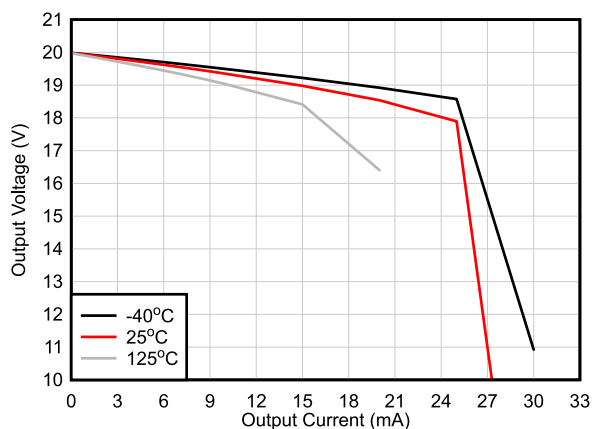
図 6-12. 出力電圧スイングと出力電流との関係 (ソース)
