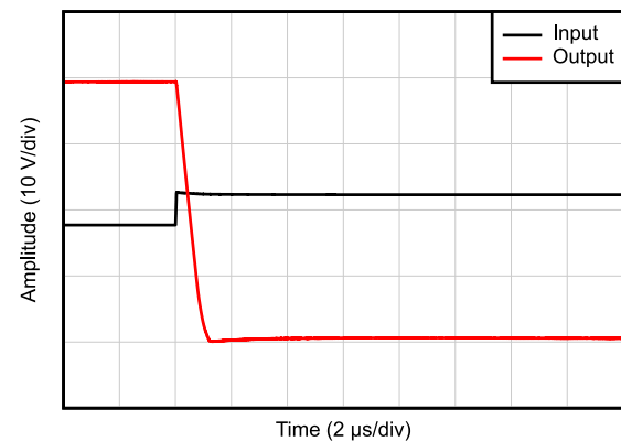
図 6-30. 負の過負荷からの回復
