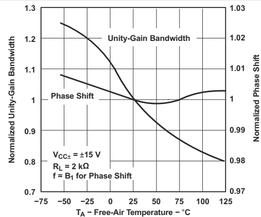
図 6-49. 正規化されたユニティ・ゲイン帯域幅および位相シフトと自由気流温度との関係
