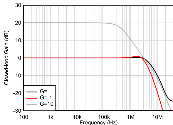
図 6-9. 閉ループ・ゲインと周波数との関係
