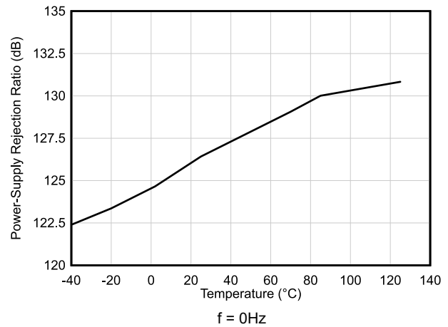
図 6-16. PSRR と温度との関係 (dB)
