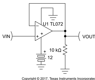
図 9-3. 単一電源のユニティ・ゲイン・アンプ
