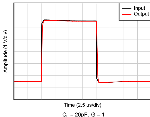
図 6-35. 大信号ステップ応答
