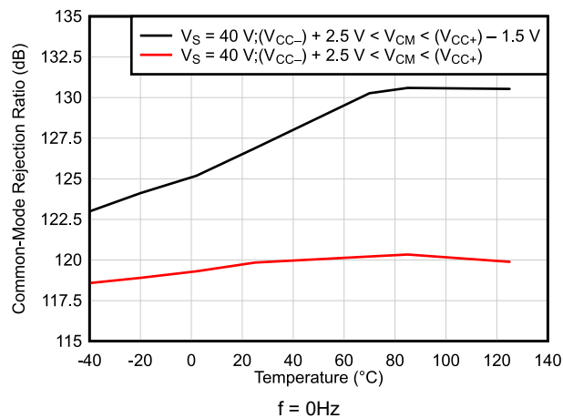
図 6-15. CMRR と温度との関係 (dB)
