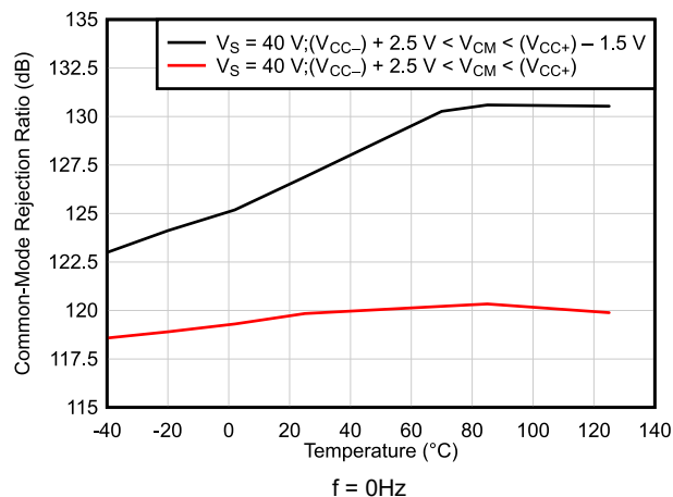
図 6-15. CMRR と温度との関係 (dB)
