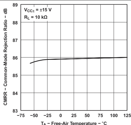
図 6-50. 同相信号除去比と自由気流温度との関係
