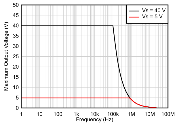
図 6-37. 最大出力電圧と周波数との関係
