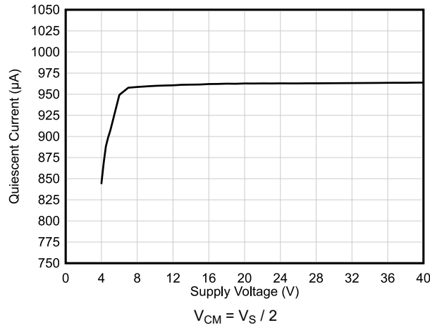
図 6-21. 静止電流と電源電圧との関係
