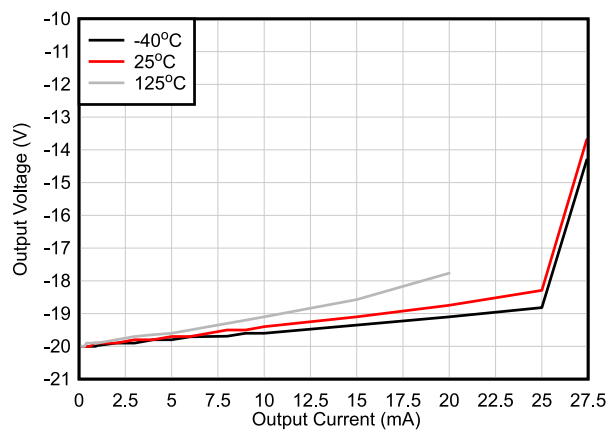
図 6-13. 出力電圧スイングと出力電流との関係 (シンク)
