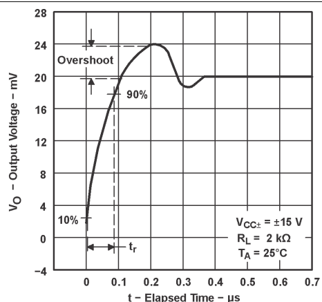
図 6-58. 出力電圧と経過時間との関係
