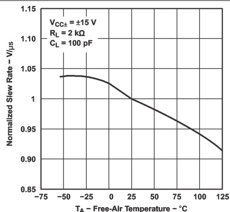
図 6-54. 正規化されたスルーレートと自由気流温度との関係
