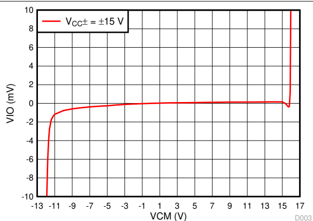
図 6-59. V_{IO} と V_{CM} との関係
