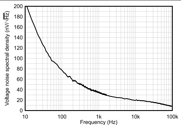
図 6-18. 入力電圧ノイズ・スペクトル密度と周波数との関係
