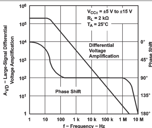
図 6-48. 大信号の差動電圧増幅および位相シフトと周波数との関係
