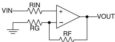
図 9-11. 非反転構成のオペアンプの回路図
