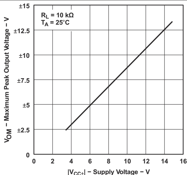
図 6-46. 最大ピーク出力電圧と電源電圧との関係
