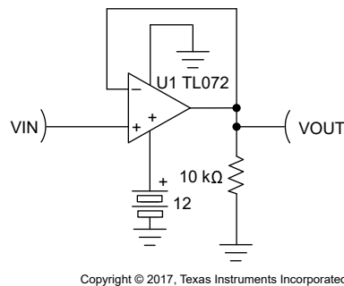
図 9-3. 単一電源のユニティ・ゲイン・アンプ
