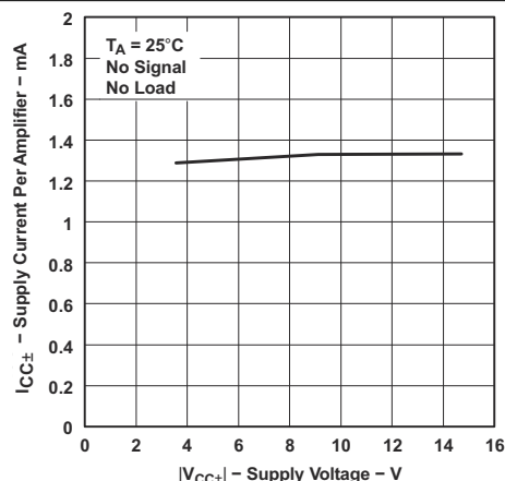
図 6-51. アンプごとの電源電流と電源電圧との関係
