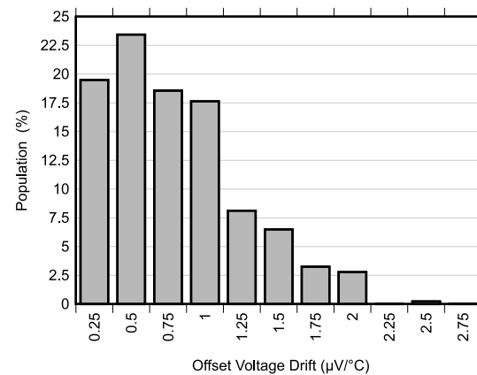
図 6-2. オフセット電圧ドリフトの分布
