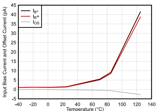
図 6-11. 入力バイアス電流と温度との関係
