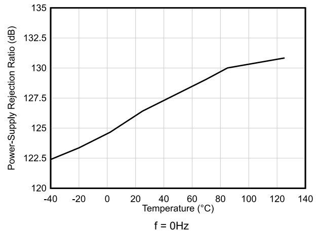
図 6-16. PSRR と温度との関係 (dB)
