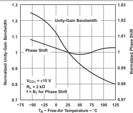
図 6-49. 正規化されたユニティ・ゲイン帯域幅および位相シフトと自由気流温度との関係
