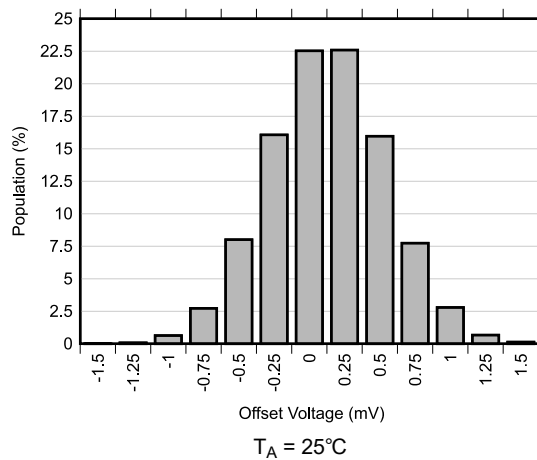
図 6-1. オフセット電圧の製品分布
