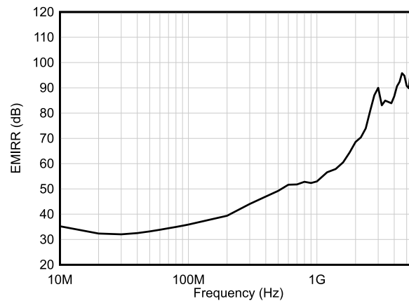
図 6-39. EMIRR (電磁干渉除去比) と周波数との関係
