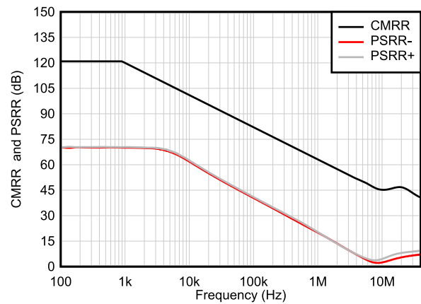
図 6-14. CMRR および PSRR と周波数との関係
