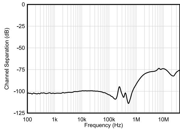
図 6-38. チャンネル・セパレーションと周波数との関係
