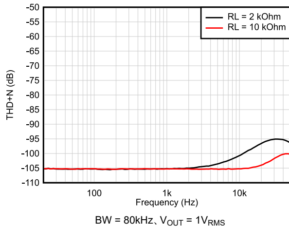
図 6-19. THD+N 比と周波数との関係
