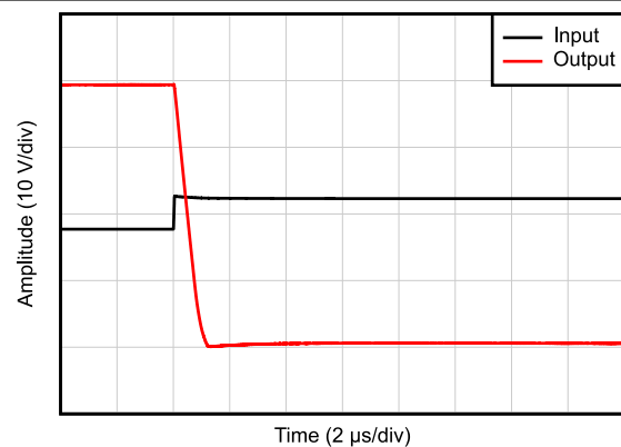
図 6-30. 負の過負荷からの回復
