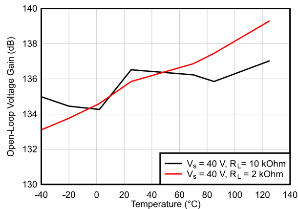
図 6-23. 開ループ電圧ゲインと温度との関係 (dB)
