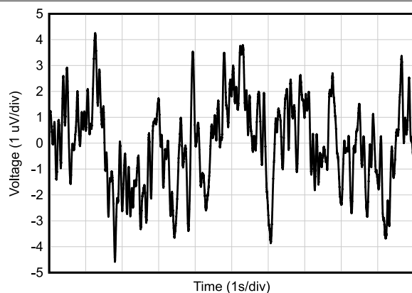
図 6-17. 0.1Hz~10Hz のノイズ
