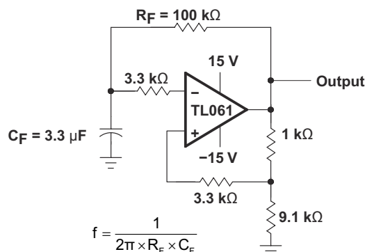
図 9-4. 0.5-Hz Square-Wave Oscillator
