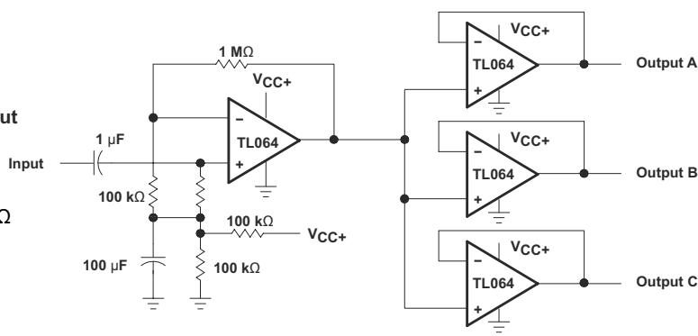
図 9-6. Audio-Distribution Amplifier
