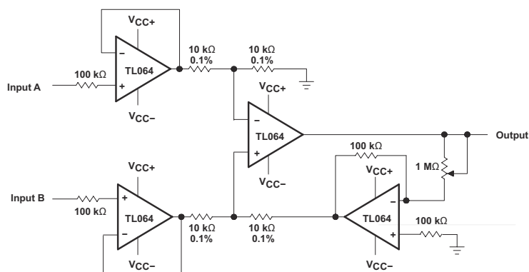
図 9-3. Instrumentation Amplifier
