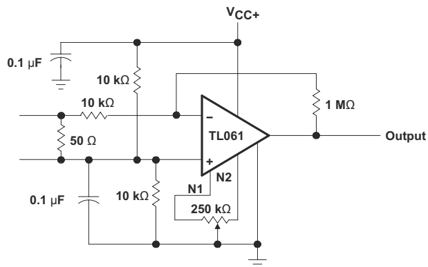
9-8. AC Amplifier
