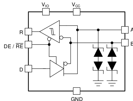
THVD14x9V のブロック図
