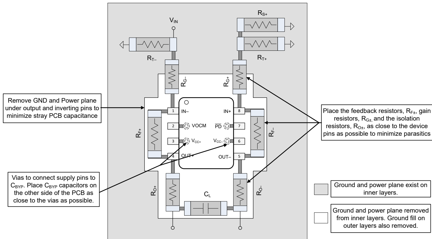
图 9-9. Layout Recommendations
