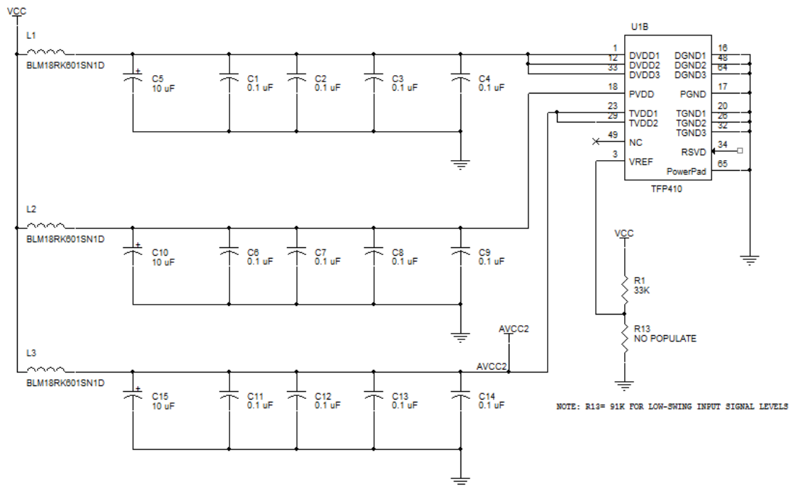
图 7-3. Power Decoupling
