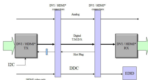
代表的な HDMI インターフェイス
