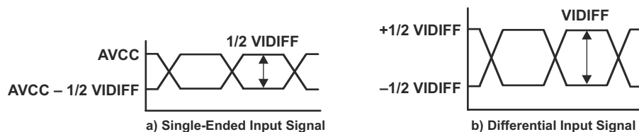
FIG 7-2. TMSD Inputs
