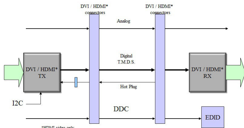
TFP401 概念図
