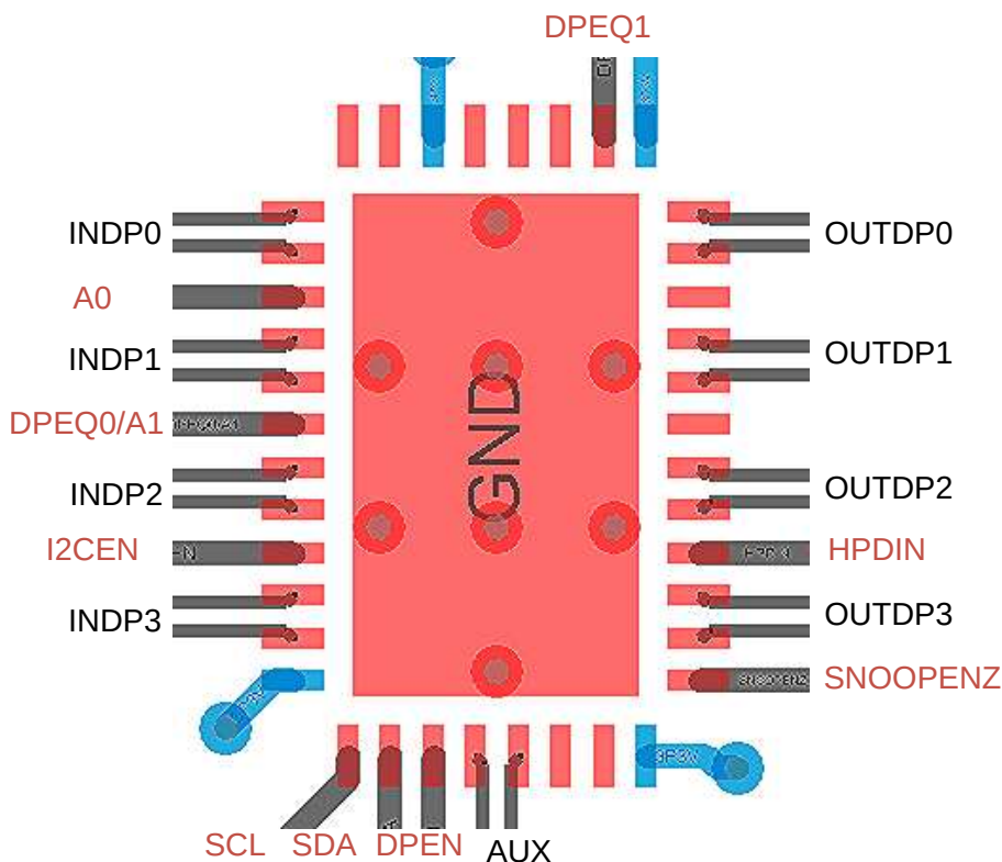
图 21. Layout Example
