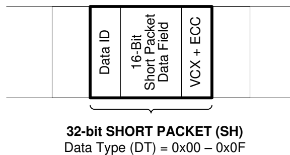
図 7-7. CSI-2 Short Packet Structure
