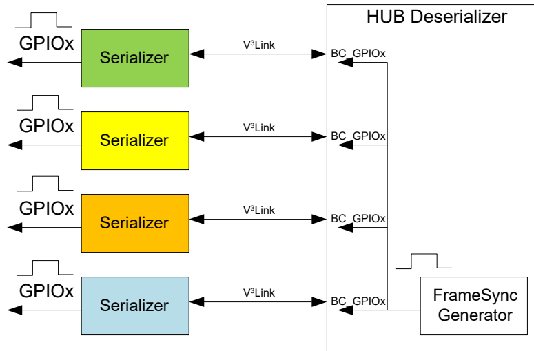
図 7-16. Internal FrameSync
