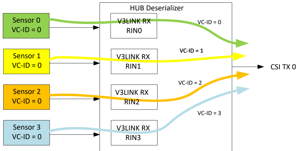
図 7-10. VC-ID Mapping Example 1
