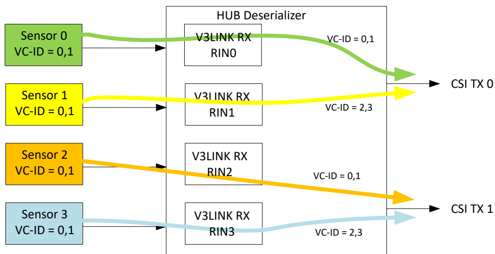
図 7-11. VC-ID Mapping Example 2
