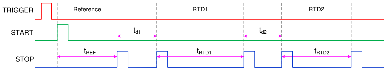
図 8-11. 温度測定の出カコック
