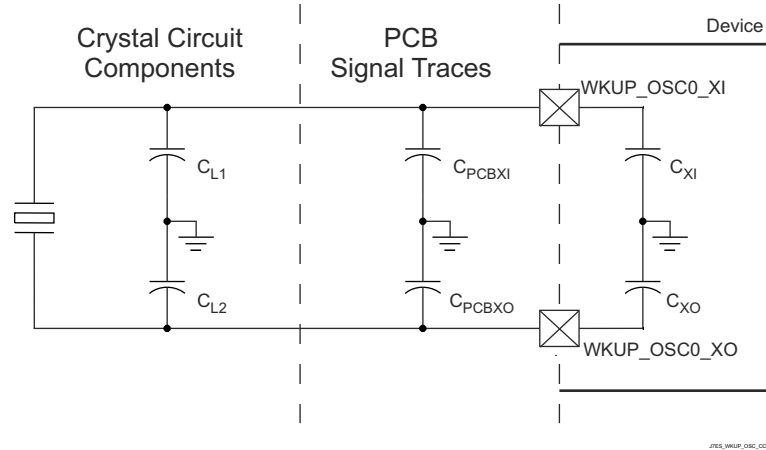
図 6-25. Load Capacitance
