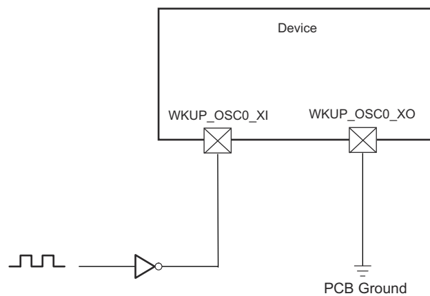
図 6-27. 1.8-V LVC MOS-Compatible Clock Input
