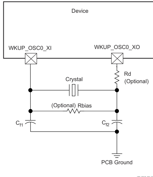
図 6-23. WKUP_OSC0 Crystal Implementation
