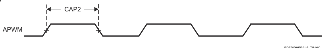
図 6-45. eCAP の出力タイミング
