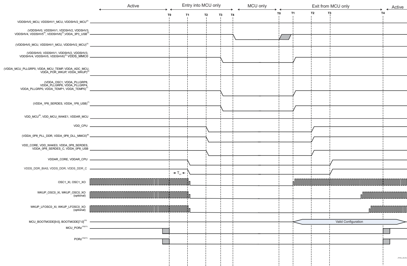
図 6-7. 独立した MCU およびメイン ドメイン、MCU のみ状態への移行および復帰シーケンス
