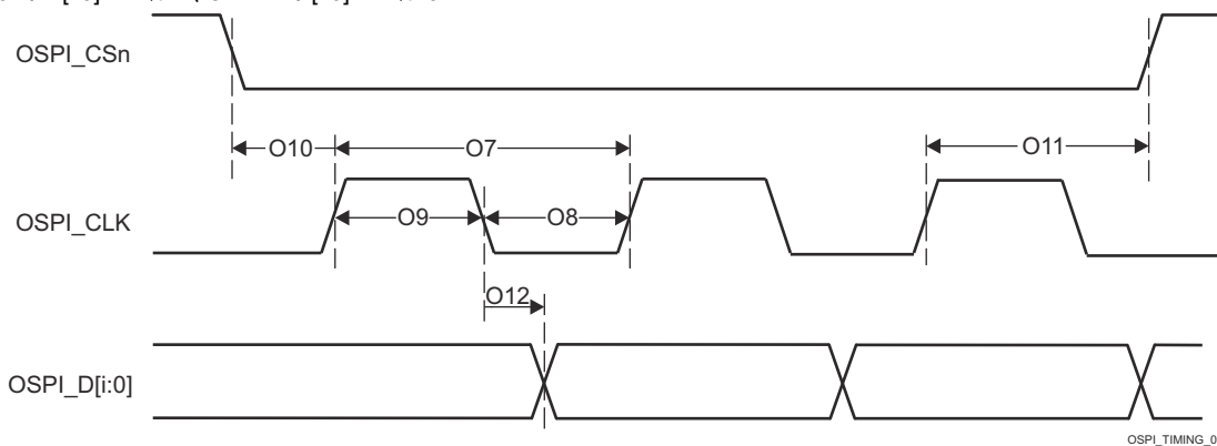
図 6-104. OSPI のスイッチング特性 – SDR
