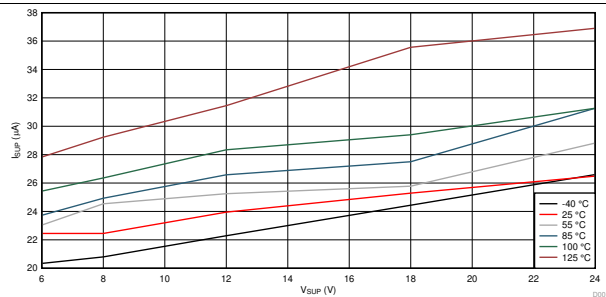
図 1. I_{SUP} vs V_{SUP} Sleep Mode
