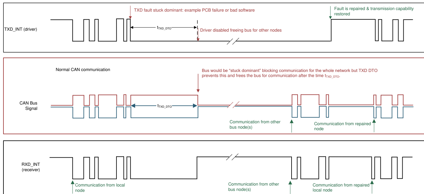
图 24. Example timing diagram with TXD_INT DTO
