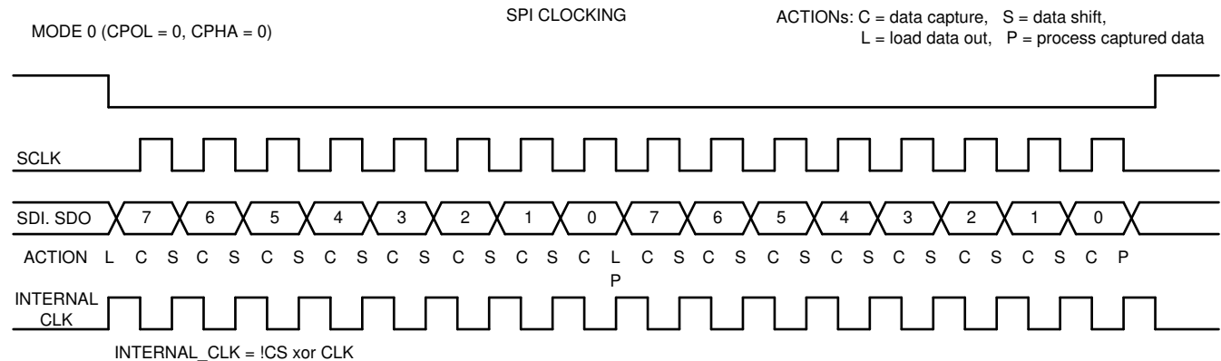
図 34. SPI Clocking
