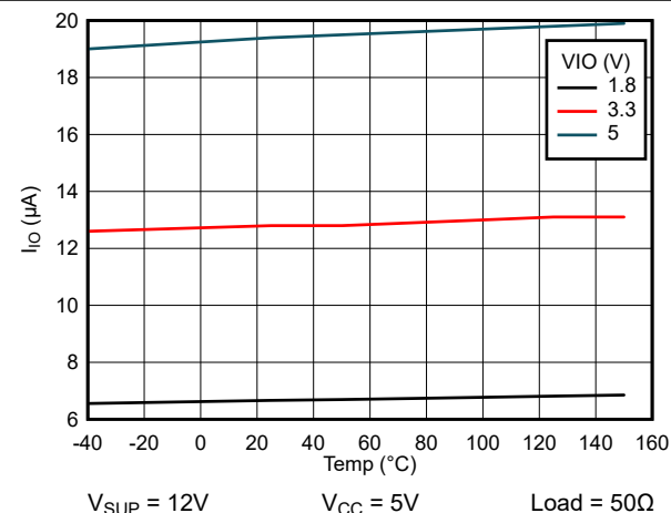
図 6-6. Normal Mode Dominant: I_{IO} vs Temperature
