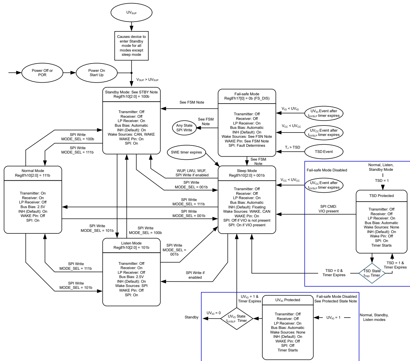
图 8-10. TCAN1465-Q1 Device State Diagram
