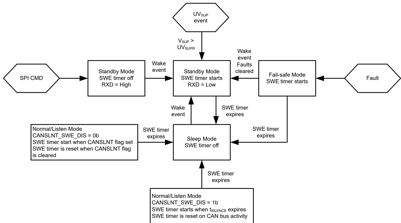
図 8-23. Sleep Wake Error (SWE) Timer if Enabled
