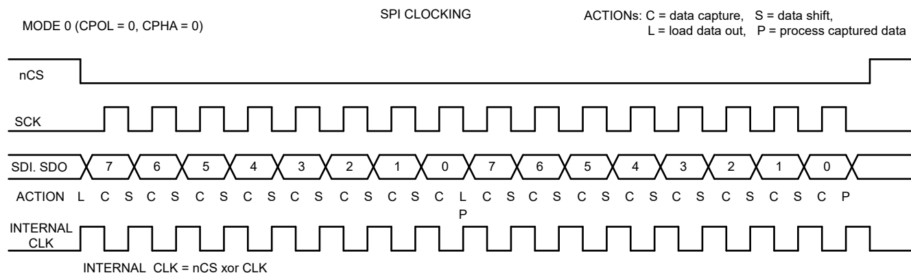
図 8-40. SPI Clocking
