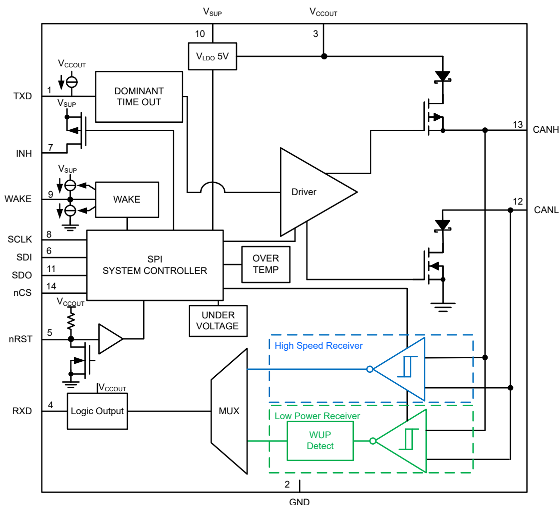
9-1. TCAN1167-Q1
