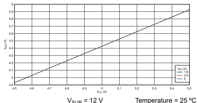
8-2. VOD vs VCC
