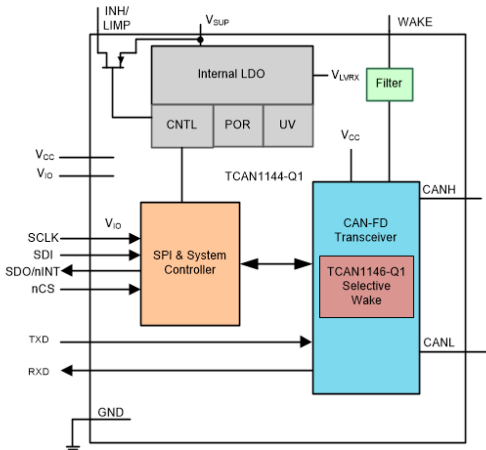
FIG 10-2. TCAN1144-Q1 and TCAN1146-Q1 Functional Block Diagram
