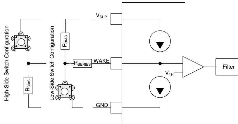
図 8-6. TCAN1043xx-Q1 WAKE Circuit Example
