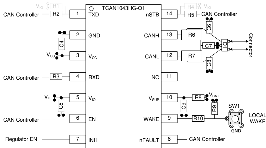
9-6. TCAN1043xx-Q1 Layout Example
