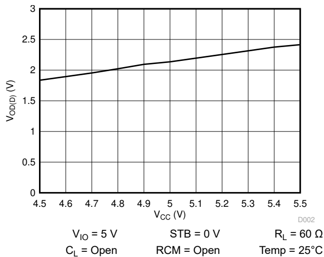
7-2. V_{OD(D)} over V_{CC}
