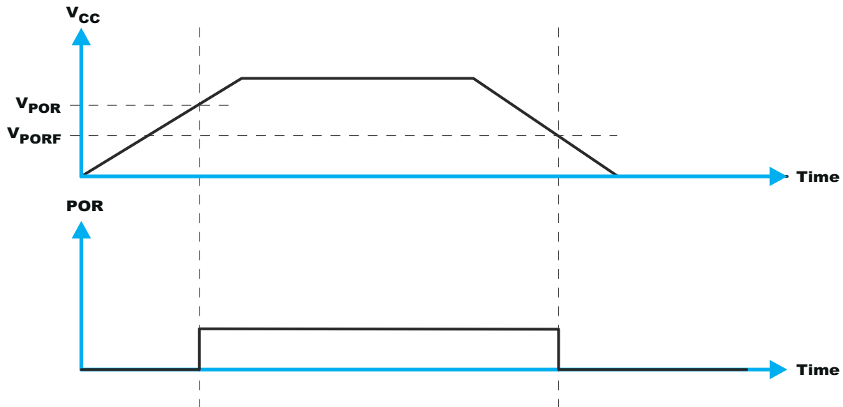
FIG 9-9. V_{POR}
