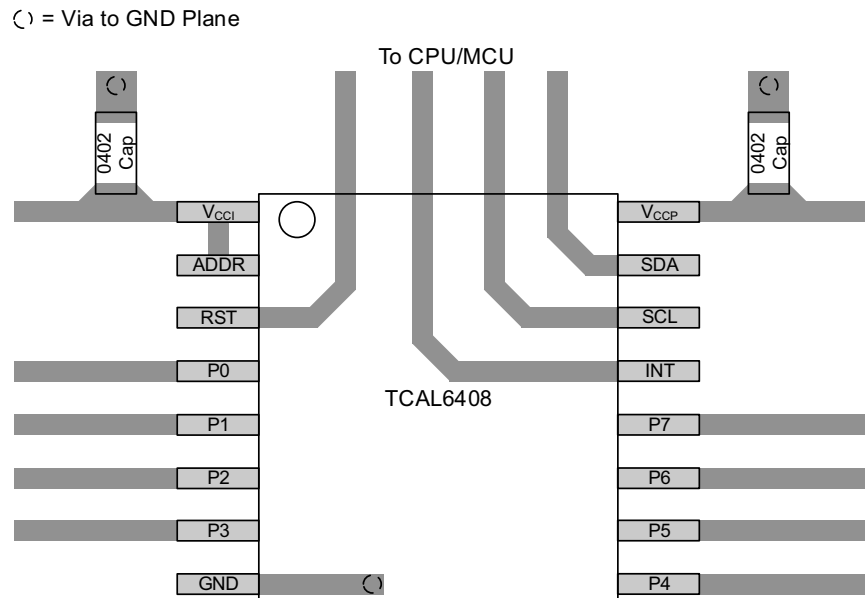
図 8-10. TCAL6408 のレイアウト
