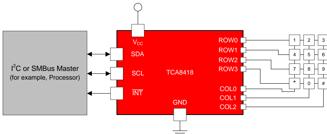
概略回路図
