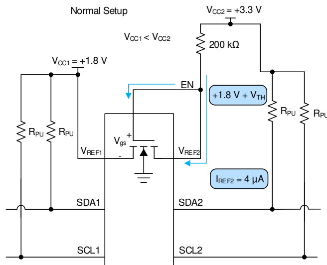
図 7-1. Normal Setup
