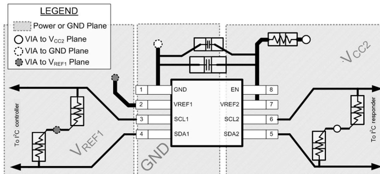
図 8-8. Layout Example
