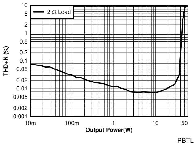
7-37. THD+N vs Power - PBTL - 384kHz
