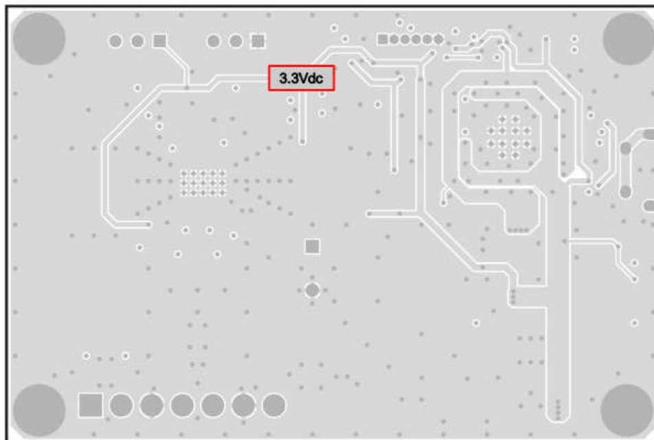
図 10-3. Power Layer
