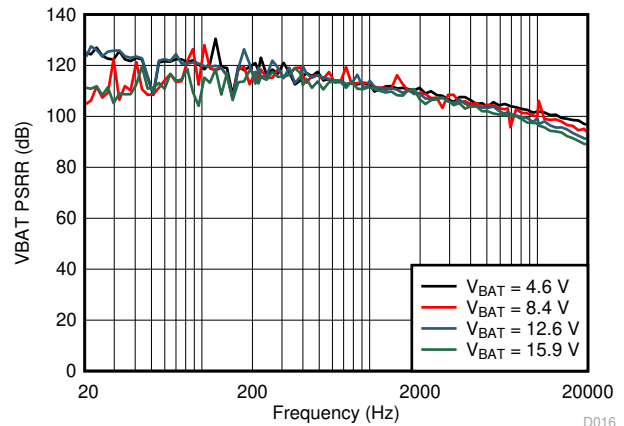
图 6-16. VBAT PSRR vs Frequency
