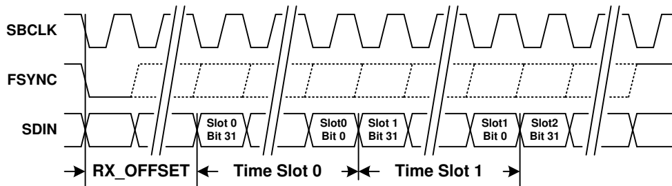
図 8-9. TDM RX Time Slots
