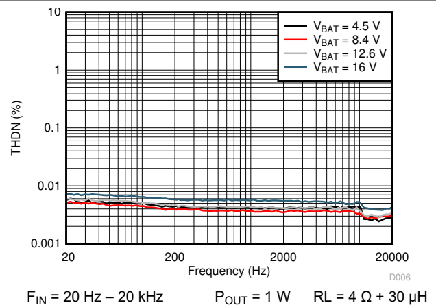
图 6-6. THD+N vs Frequency
