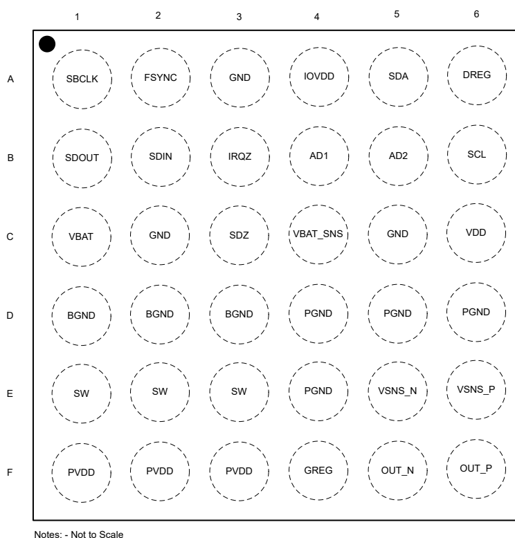
図 4-1. パッケージの上面図のピン配置
