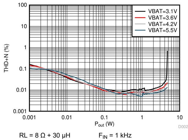
図 5-7. THD+N vs Output Power (DSBGA Package)
