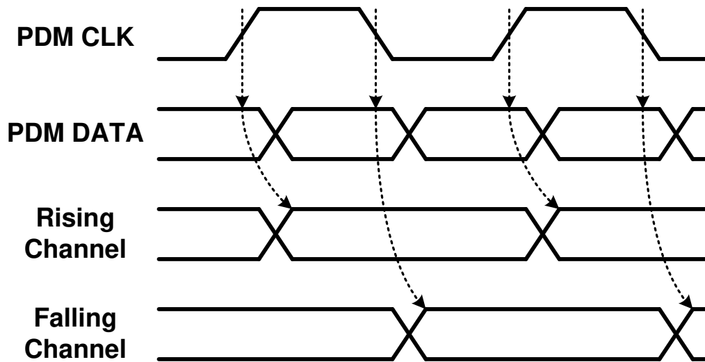
図 7-11. PDM Waveform
