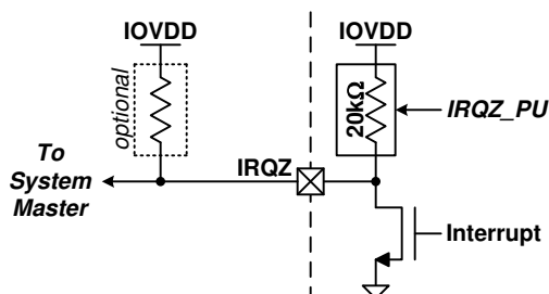
図 7-10. IRQZ Pin
