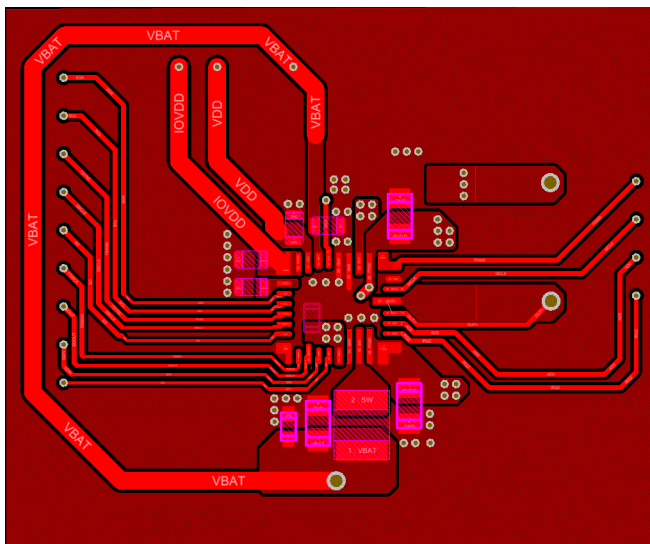
図 10-7. QFN Package Top Layer
