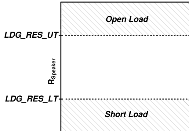
図 7-21. Load Diagnostics
