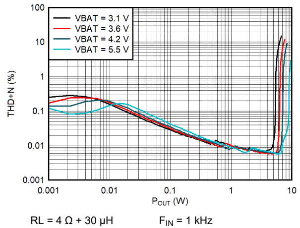
図 5-6. THD+N vs Output Power (QFN Package)
