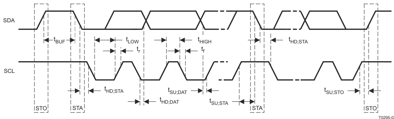
图 6-5. I 2 C 接口时序
