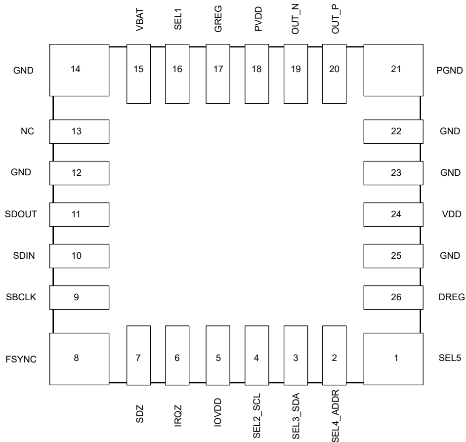
図 4-1. QFN Package Bottom View
