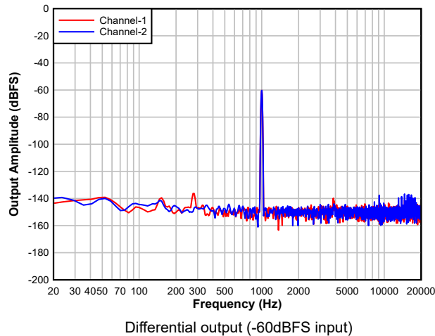
图 8-2. DAC FFT with -60dBFS Input
