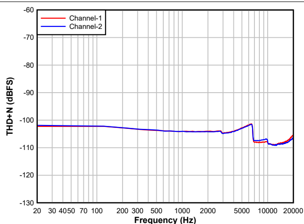
図 5-10. DAC THD+N レベル対周波数
