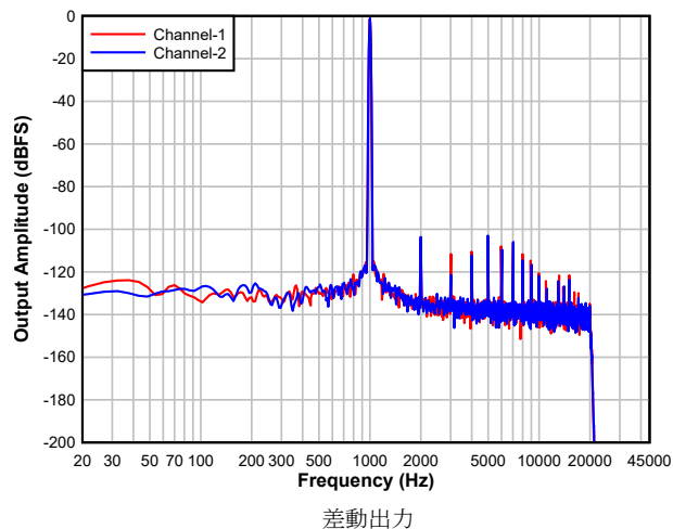
図 5-15. -1dBFS 入力の DAC FFT
