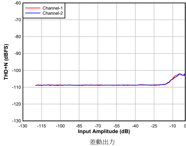
図 5-5. DAC の THD +N レベルと入力との関係
