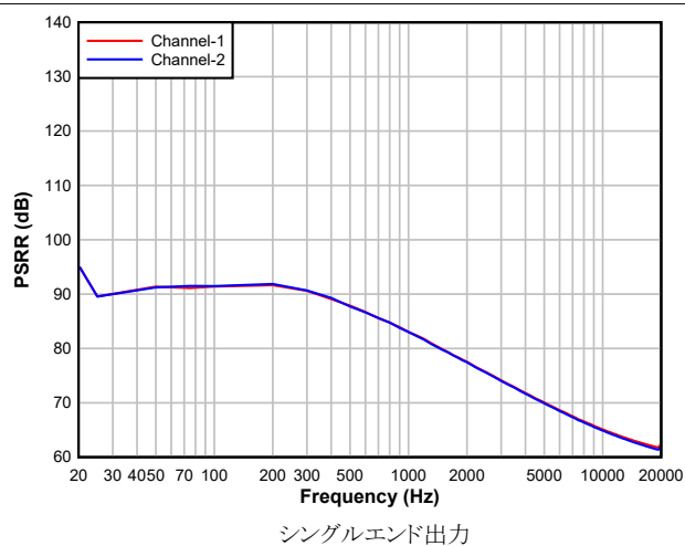
図 5-17. DAC PSRR と周波数との関係
