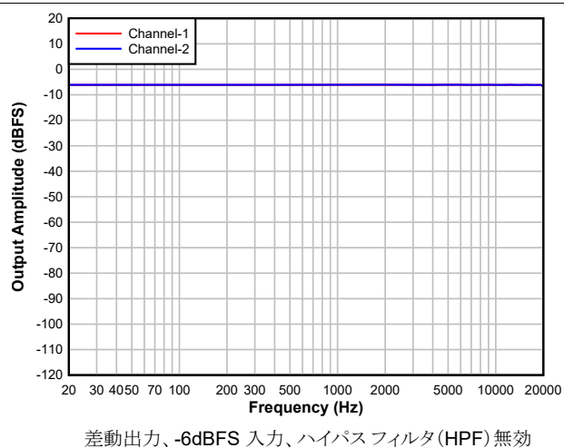
図 5-18. DAC の周波数応答
