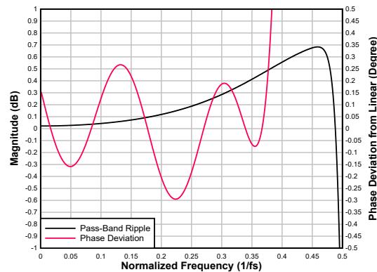
図 6-83. 低レイテンシ デシメーション フィルタのパスバンド リップルと位相偏差
