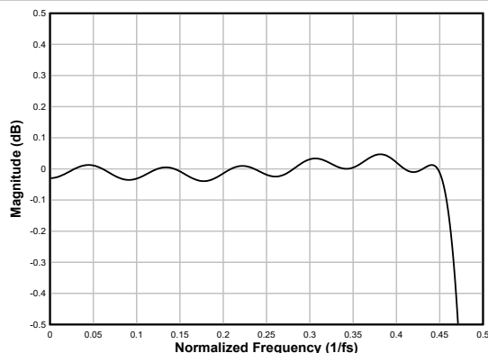
図 6-69. 線形位相デシメーション フィルタのパスバンドリップル
