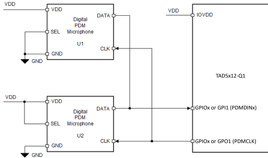
図 6-18. TAD5112-Q1 のデジタル PDM マイクの接続図
