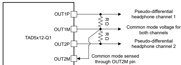
図 6-16. 外部同相モード センスを使用した擬似差動出力接続 (OUT1x_CFG[2:0] = 3'b101)
