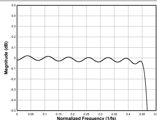
図 6-31. 線形位相補間フィルタのパスバンド リップル
