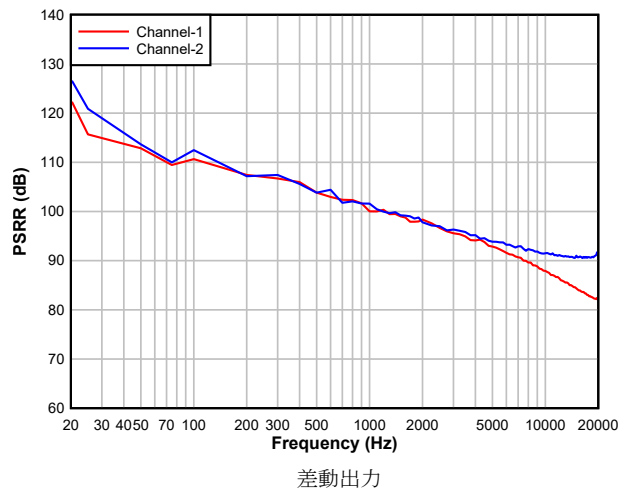
図 5-16. DAC PSRR と周波数との関係
