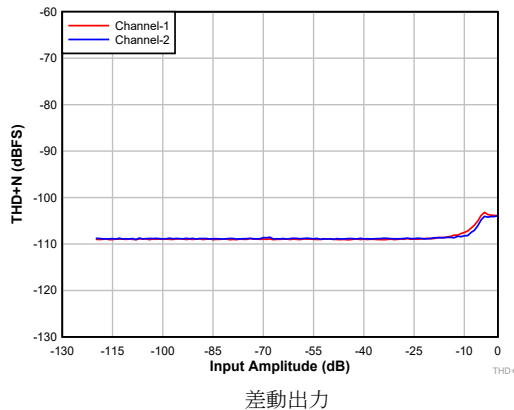
図 8-2. DAC の THD +N レベルと入力との関係
