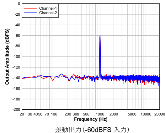
図 8-3. -60dBFS 入力の DAC FFT
