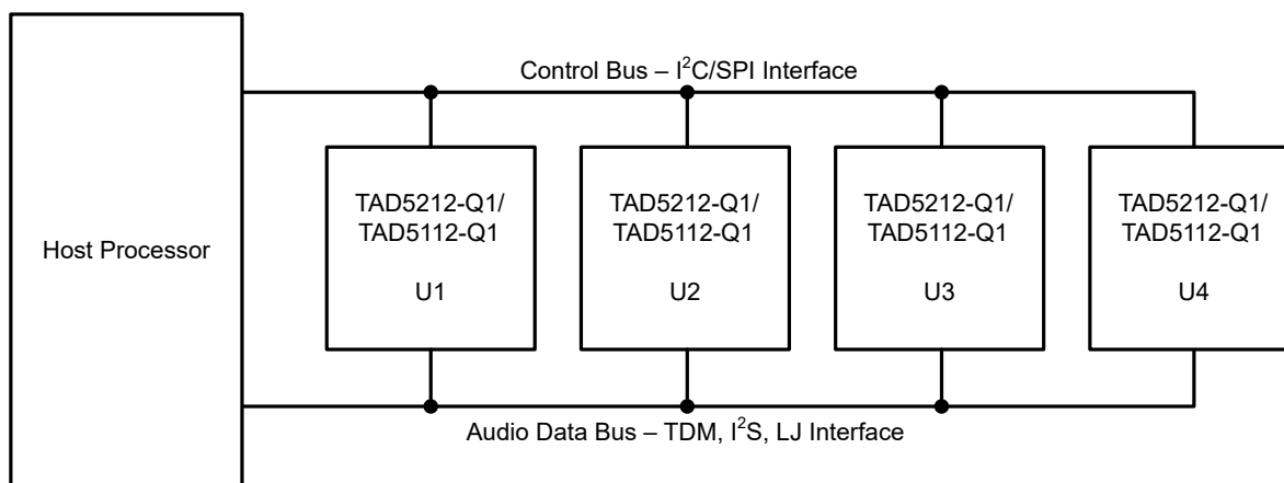
図 6-13. 制御およびオーディオ データ バスを共有する複数の TAD5112-Q1 デバイス
