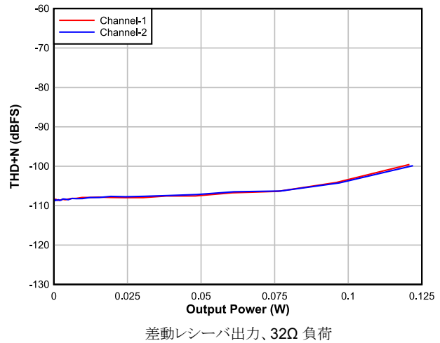
図 5-8. DAC THD+N レベルと出力パワー
