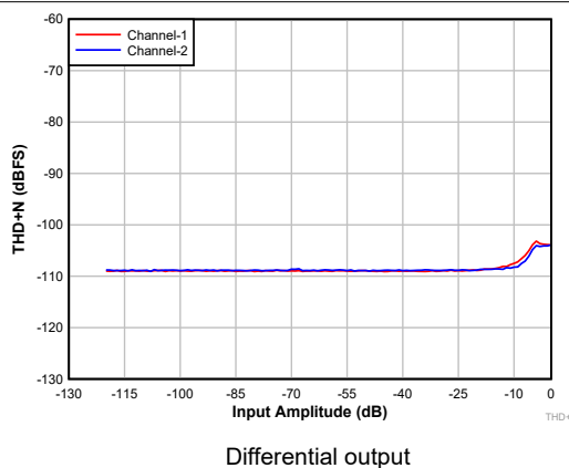
図 8-2. DAC THD+N Level vs Input
