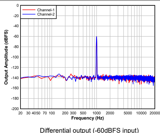
図 8-3. DAC FFT with -60dBFS Input
