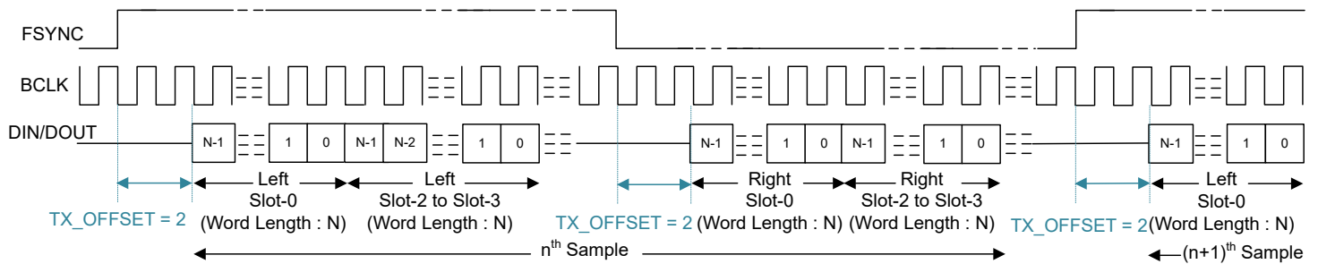
図 6-11. LJ Protocol Timing (TX_OFFSET = 2)
