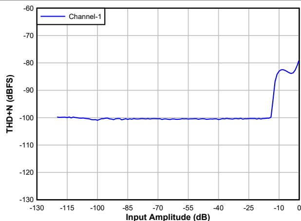
図 5-6. ADC THD+N Level vs Input
