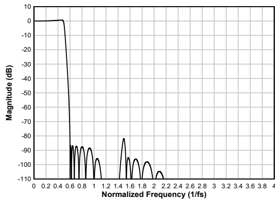
図 6-40. 低レイテンシのデシメーション フィルタの振幅応答
