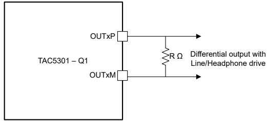
図 6-19. 差動出力接続 (OUT1x_CFG[2:0] = 3'b000)
