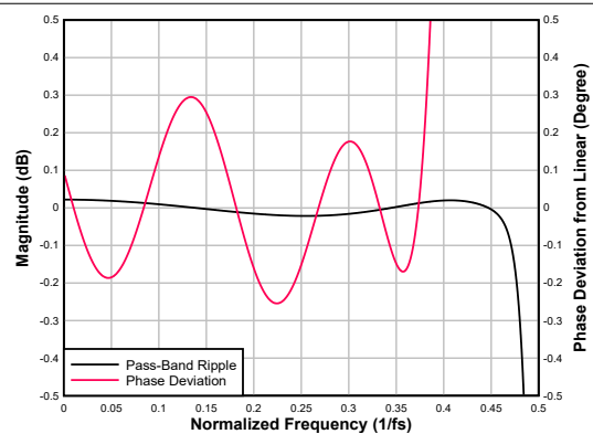
図 6-45. 低レイテンシ デシメーション フィルタのバ スバンド リップルと位相偏差
