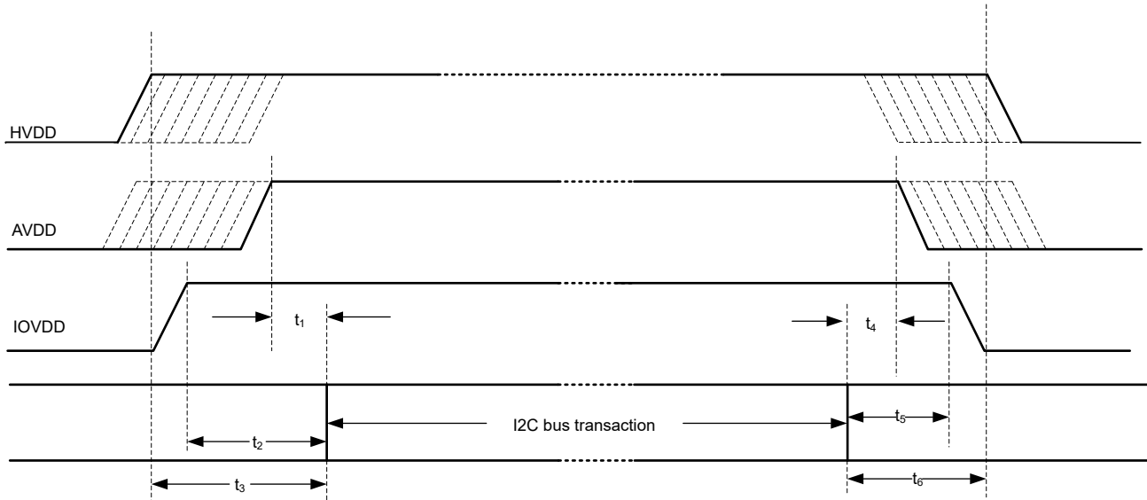
図 8-6. 電源シーケンス要件のタイミング図
