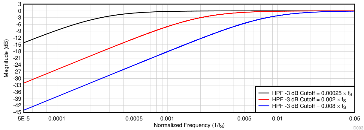
図 6-62. HPF フィルタの周波数応答プロット
