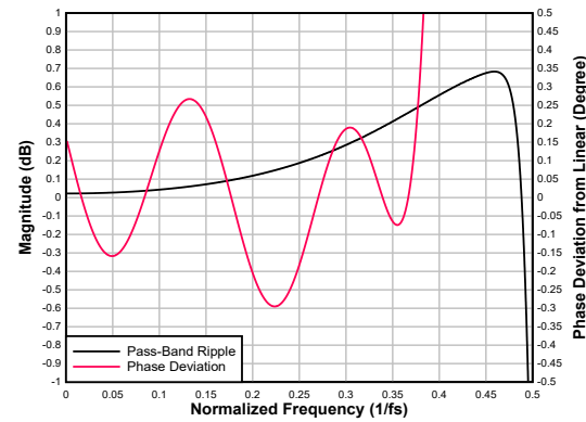
図 6-41. 低レイテンシ デシメーション フィルタのパスバンド リップルと位相偏差
