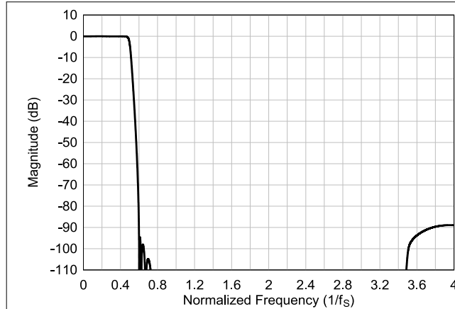
図 6-87. 超低レイテンシ補間フィルタの振幅応答
