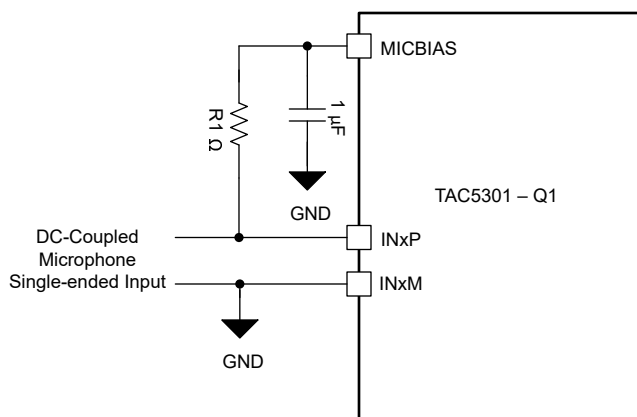
図 6-16. DC 結合マイクロフォン シングルエンド入力接続
