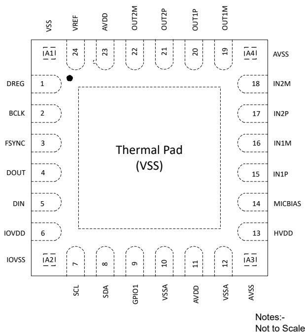
図 4-1. TAC5301-Q1 24 ピン QFN パッケージ、露出サーマルパッドおよびコーナーピン付き、上面図
