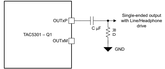
図 6-20. OUT1P でのモノ シングルエンド出力接続 (OUT1x_CFG[2:0] = 3'b010)
