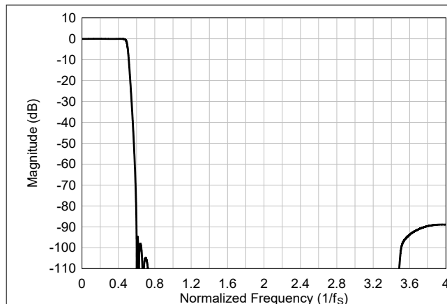
図 6-89. 超低レイテンシ補間フィルタの振幅応答
