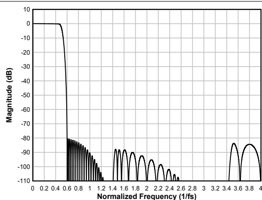
図 6-65. 線形位相補間フィルタの振幅応答
