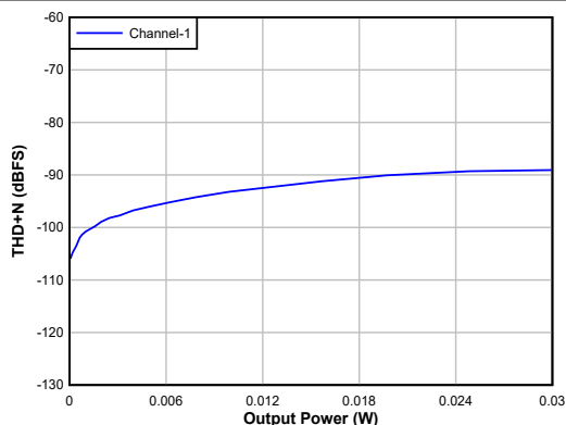
図 5-19. DAC THD+N レベルと出力パワー
