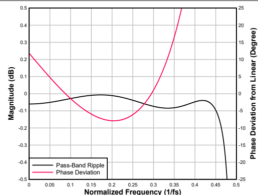
図 6-90. 超低レイテンシ補間フィルタのパス バンドリップルと位相偏差
