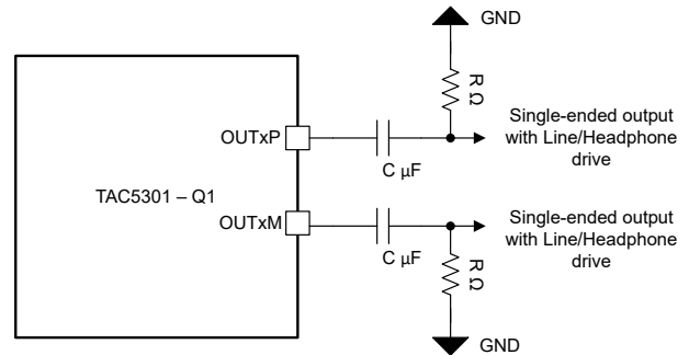
図 6-22. ステレオ シングルエンド出力接続 (OUT1x_CFG[2 : 0] = 3'b001)
