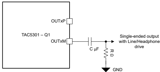
図 6-21. OUT1M でのモノ シングルエンド出力接続 (OUT1x_CFG[2:0] = 3'b011)
