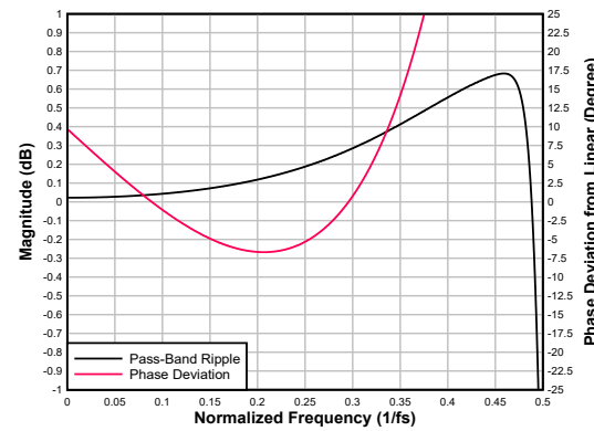
図 6-51. 超低レイテンシ デシメーション フィルタのパスバンド リップルと位相偏差
