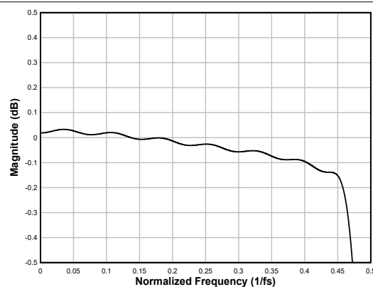
図 6-66. 線形位相補間フィルタのパスバンド リップル
