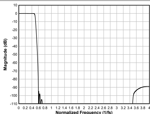
図 6-77. 低レイテンシ補間フィルタのマグニチュード 応答
