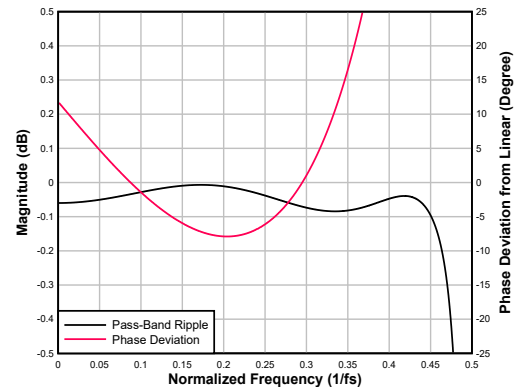
図 6-88. 超低レイテンシ補間フィルタのパス バンドリップルと位相偏差
