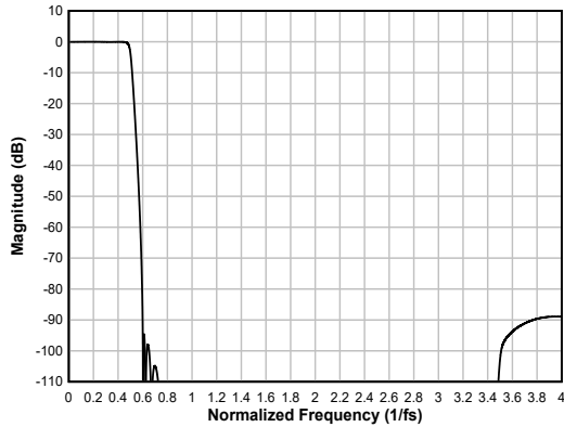
図 6-79. 低レイテンシ補間フィルタのマグニチュード応答
