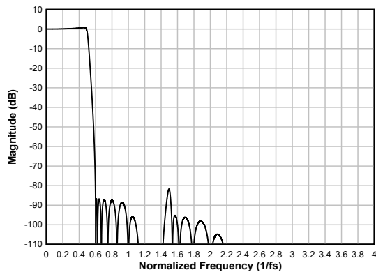
図 6-50. 超低レイテンシのデシメーション フィルタの振幅応答
