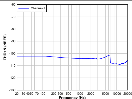
図 5-20. DAC の THD+N 比と周波数との関係
