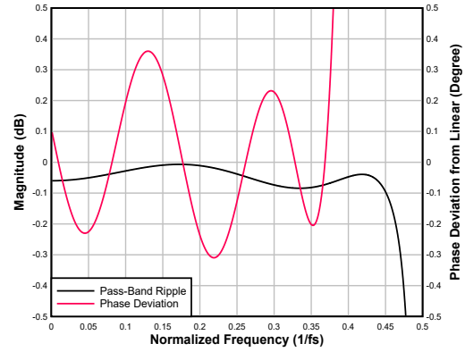
図 6-80. 低レイテンシ補間フィルタのパスバンドリップルと位相偏差
