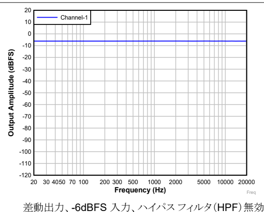
図 5-28. DAC の周波数応答
