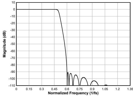
図 6-48. 低レイテンシのデシメーション フィルタの振幅応答
