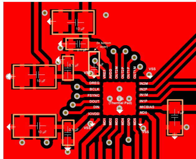
図 8-7. Example Layout
