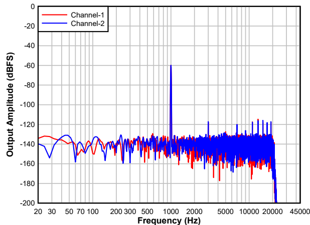
図 6-15. ADC FFT with -60dBFS Input
