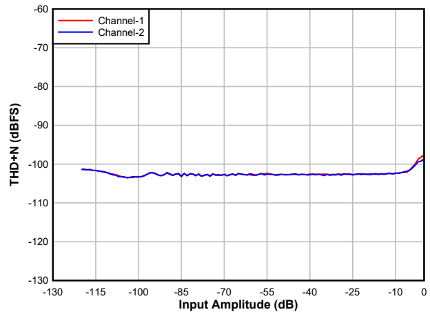
図 6-6. ADC THD+N Level vs Input
