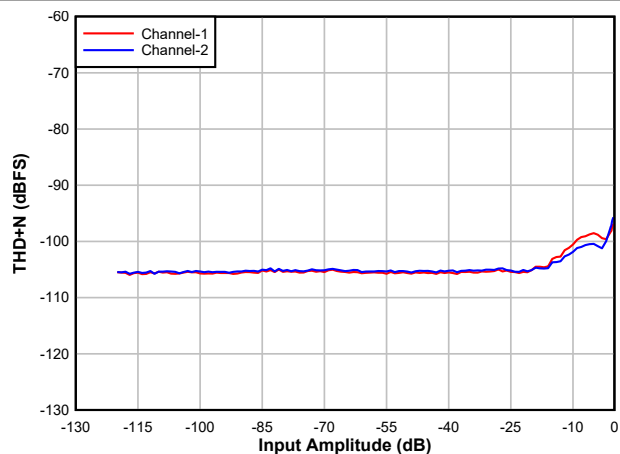
図 6-20. DAC THD+N Level vs Input
