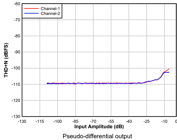
図 6-21. DAC THD+N Level vs Input
