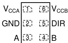
图 5-3. DRY Package Preview, 6-Pin SON (Top View)
