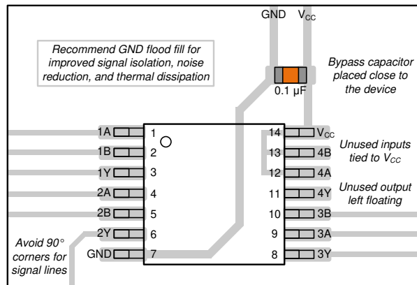
図 8-3. Example Layout for the SN74LVC7032A-Q1
