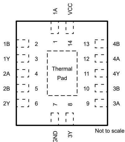
図 4-1. SN74LVC7032A-Q1 BQA Package, 14-Pin WQFN (Top View)
