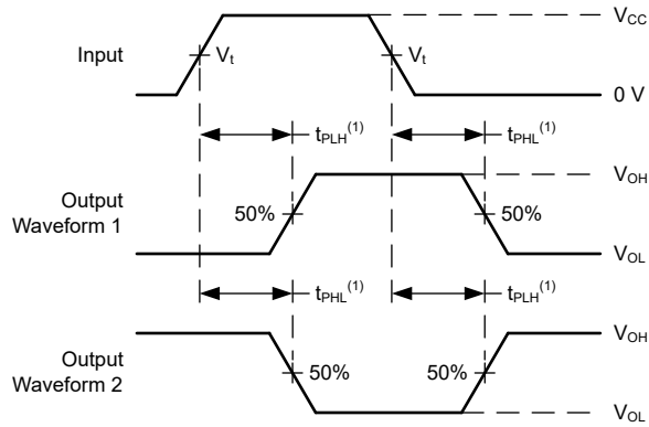
図 6-3. 電圧波形、伝搬遅延
