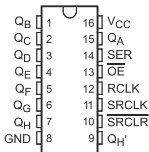
図 4-1. PW パッケージ 16 ピン TSSOP (上面図)
