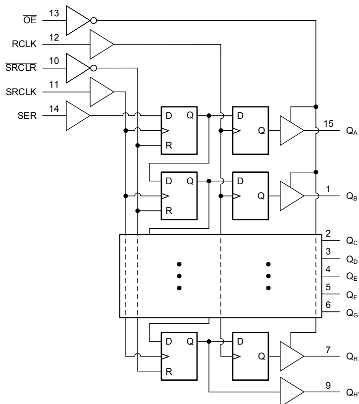
図 7-1. SN74LVC595A の論理図 (正論理)
