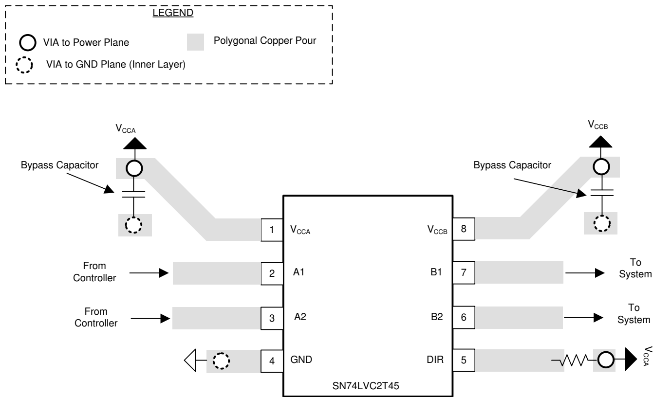
図 8-3. SN74LVC2T45 Layout Example
